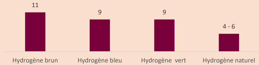
Graphique. TRL des différentes techniques de production/extraction de l'hydrogène.
